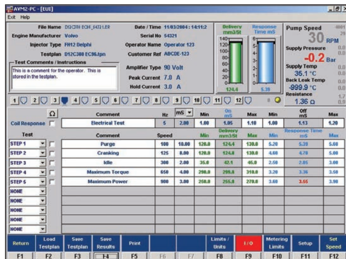
Figure 1 Banc d'essai AVM2-PC, écran d'essai d'injecteur EUI.
